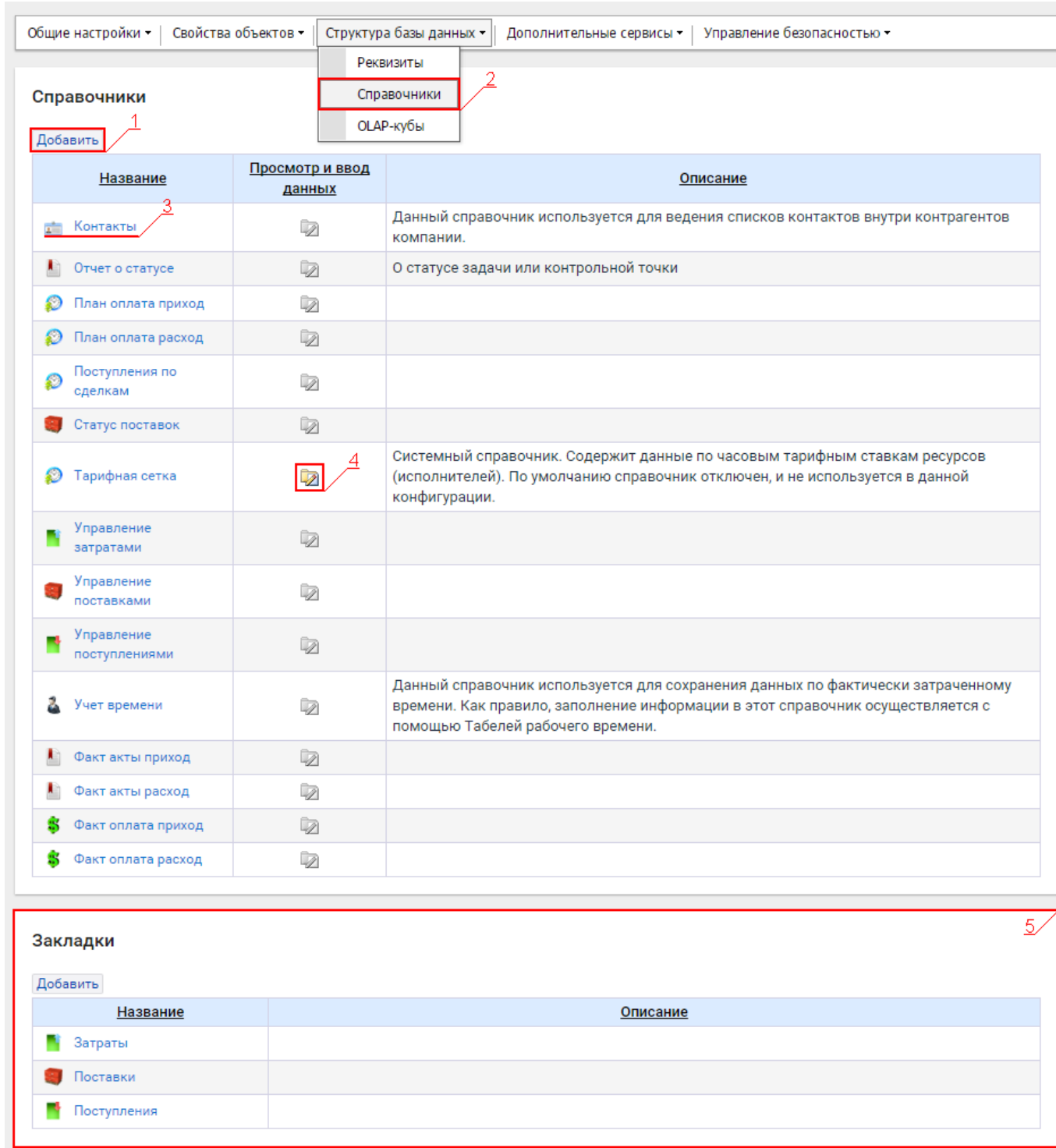
Рисунок 1 – Список справочников
