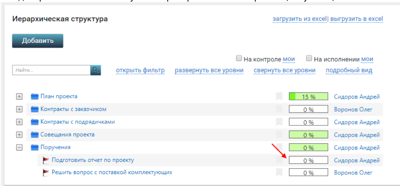
Рисунок 2 – Иерархическая структура
