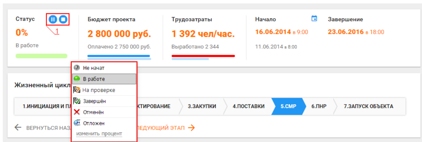
Рисунок 1 - Статусы проекта
