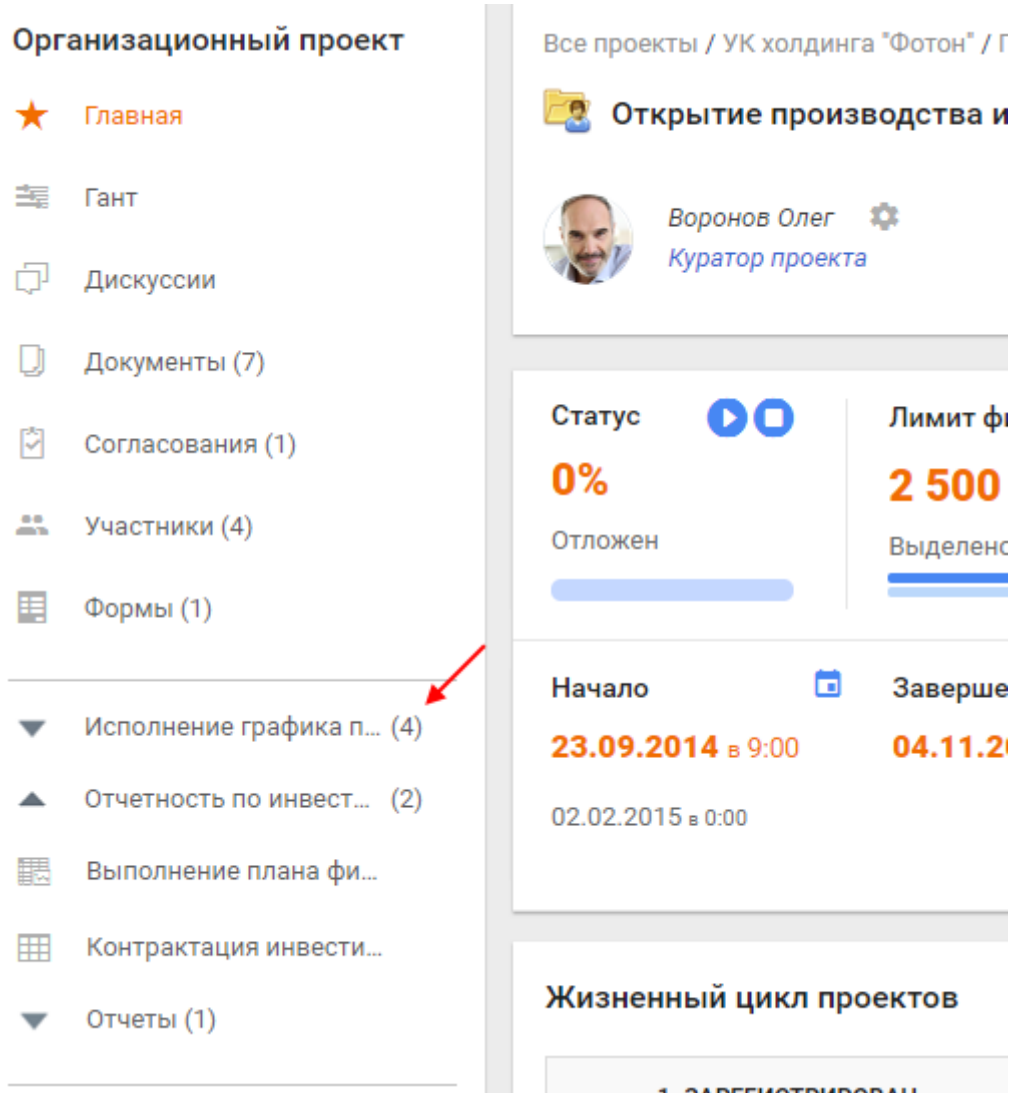
Рисунок 4 – Сгруппированные отчеты
