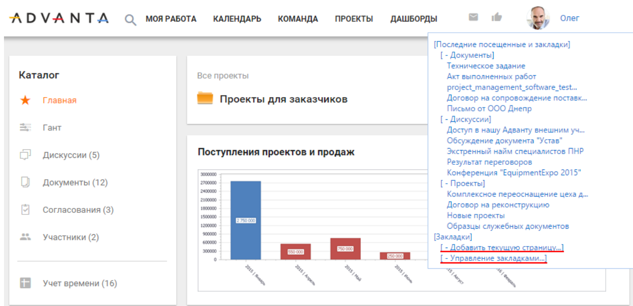
Рисунок 1 – Управление закладками
