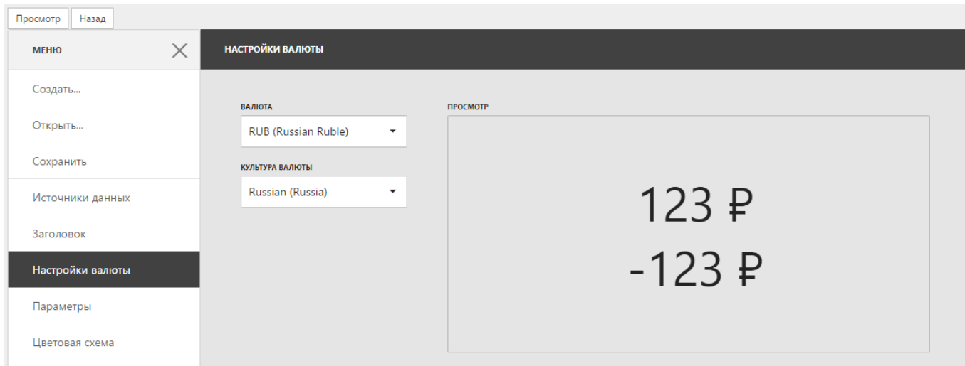
Рисунок 8 - Выбор валюты
