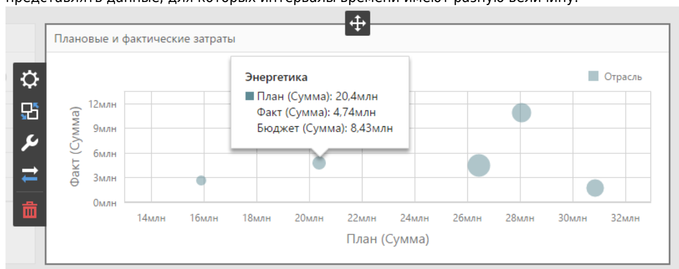
Рисунок 6 – Точечная диаграмма
