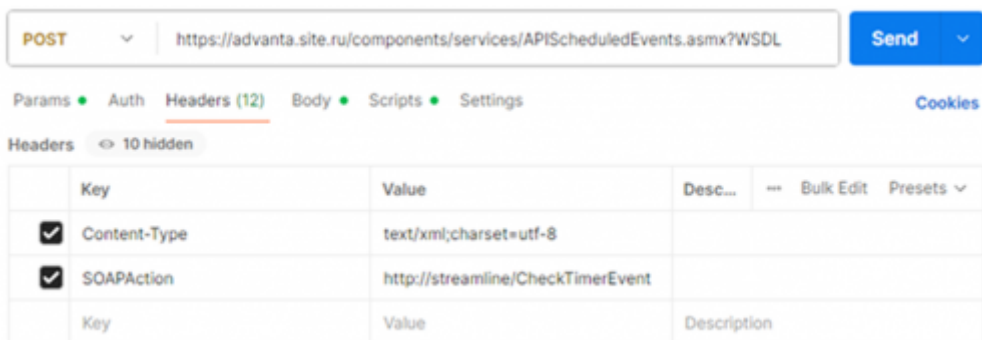
Рисунок 10. Настройки заголовков вызова API «CheckTimerEvent»
