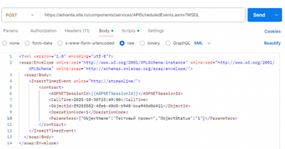
Рисунок 7. Настройки тела запроса (закладка «Body»)
