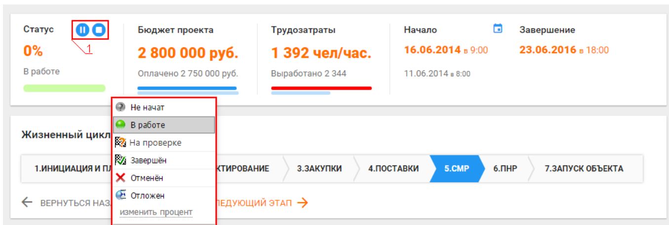
Рисунок 1 - Статусы проекта
